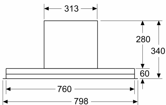
Wymiary w mm Widok z przodu
