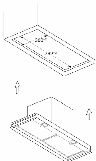
Wymiary w mm Przykład montażu w wycięciu w zabudowie meblowej
