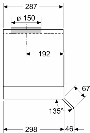
Wymiary w mm Widok z boku
