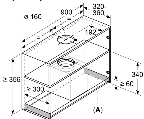
Wymiary w mm Przykładowy montaż
