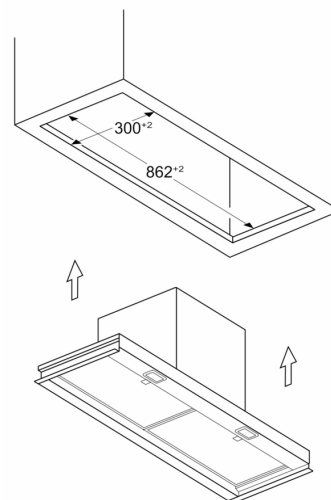
Wymiary w mm Przykład montażu w wycięciu w zabudowie meblowej
