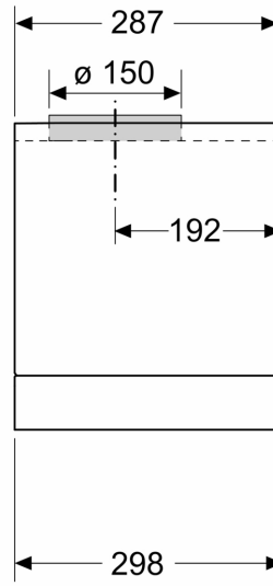
Wymiary w mm Widok z boku
