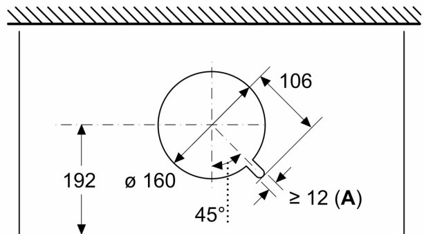
Wymiary w mm Widok z góry
