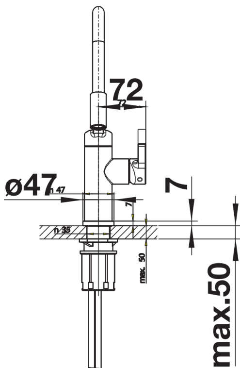
Dźwignia 2D, widok z boku
