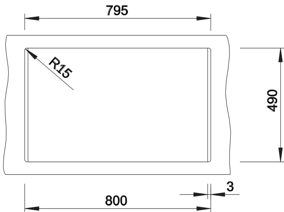
Wycięcie
