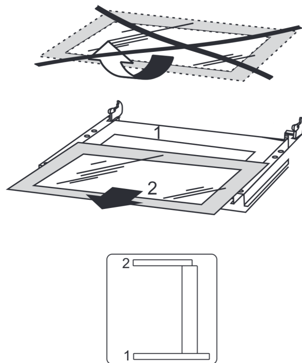
Wyjmowanie szyb wewnętrznych. 2 szyby.
