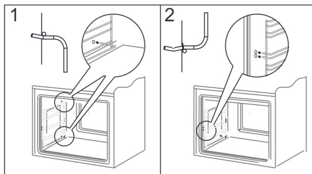
Zakładanie drabinek
