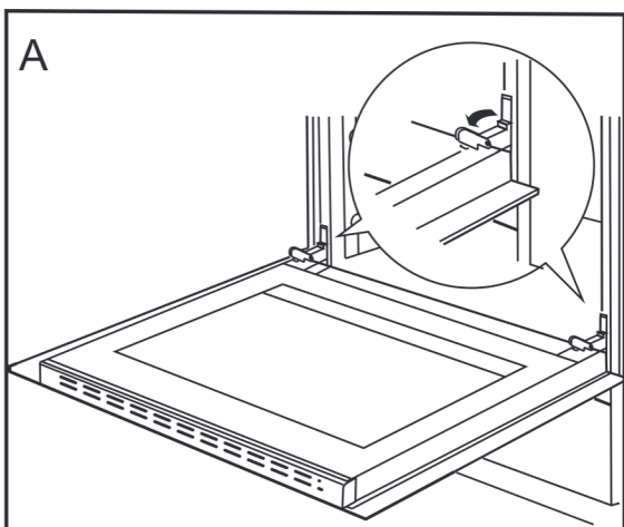
Odchylenie zabezpieczeń zawiasów
