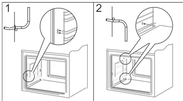
Wyjmowanie drabinek
