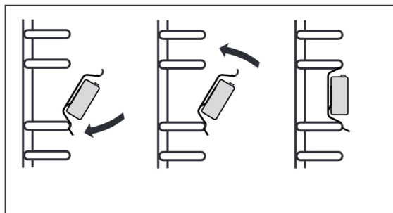
Zakładanie prowadnic teleskopowych
