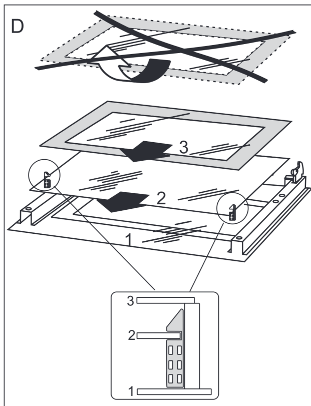
Wyjmowanie szyb wewnętrznych. 3 szyby.
