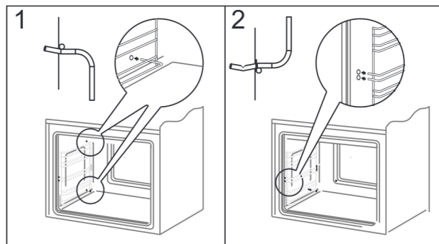
Zakładanie drabinek
