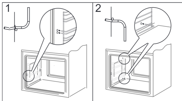
Wyjmowanie drabinek
