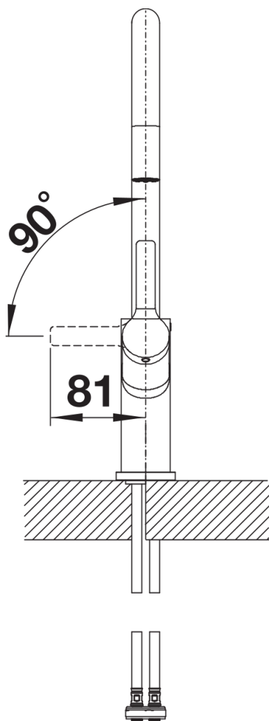
Dźwignia 2D, widok z boku
