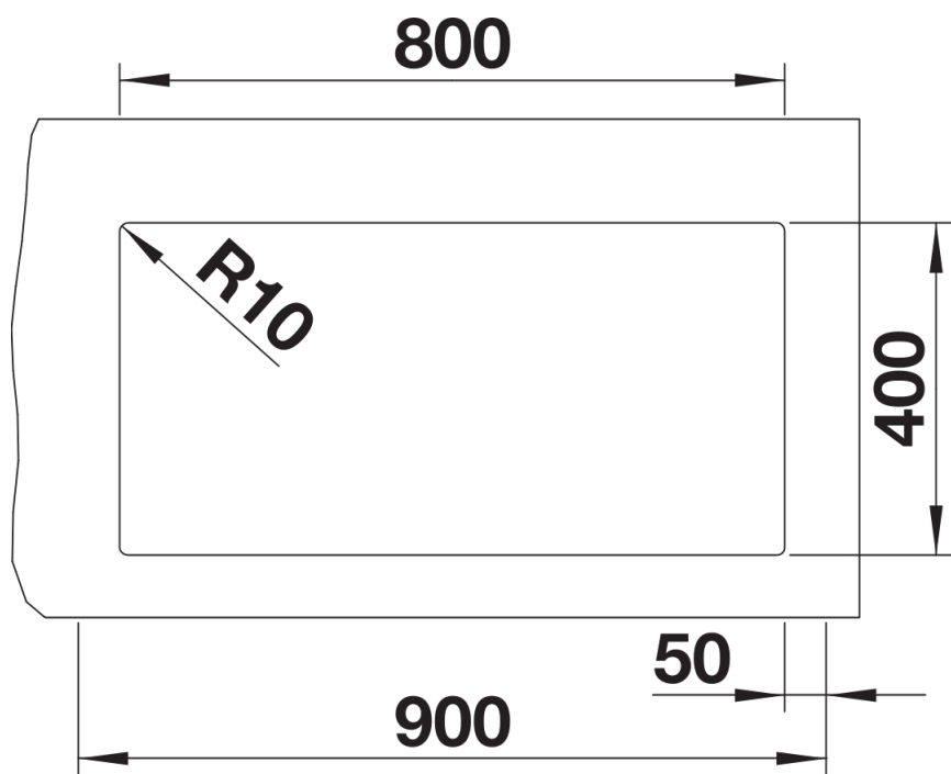
Wycięcie
