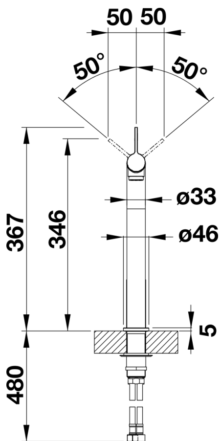
Dźwignia 2D, widok z boku
