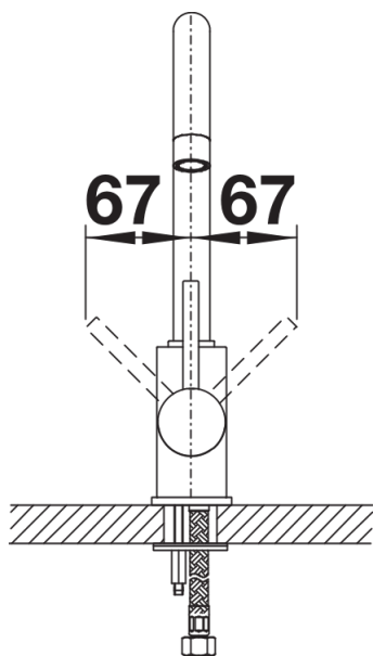
Dzwignia 2D, widok z boku
