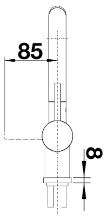
Dźwignia 2D, widok z boku
