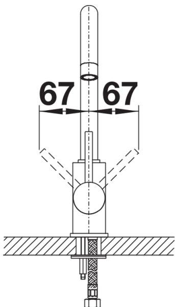
Dźwignia 2D, widok z boku
