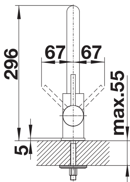
Dźwignia 2D, widok z boku
