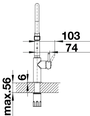
Dźwignia 2D, widok z boku
