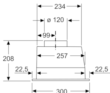
wymiary w mm
