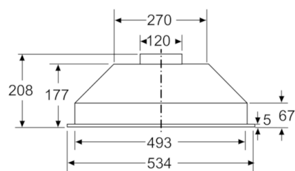
wymiary w mm
