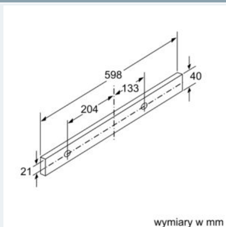
Rysunki wymiarowe
