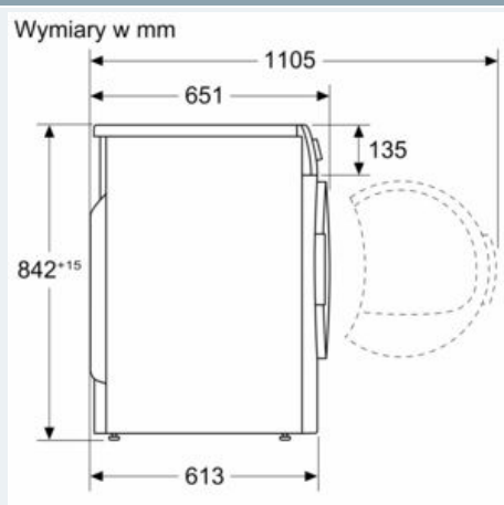
Rysunki wymiarowe
