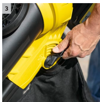
3 Dźwignia do wyboru zastosowań
